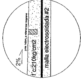
DETALLE DE ACERA
